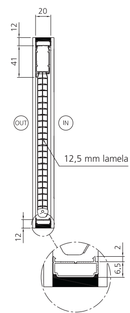
Extrudovaný "U" rámeček 20 x 6.5 mm
