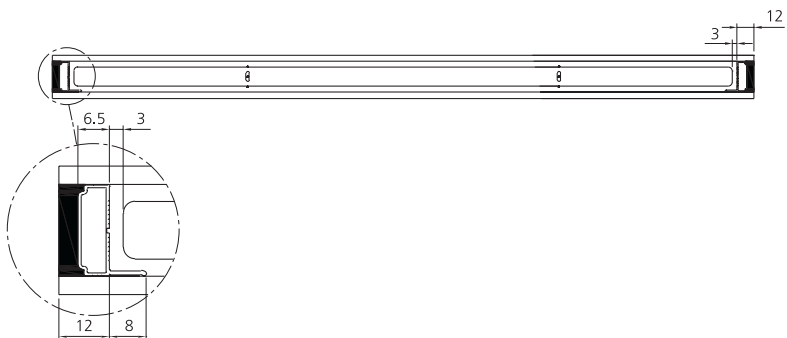
Extrudovaný "L" rámeček 20 x 6.5 mm
