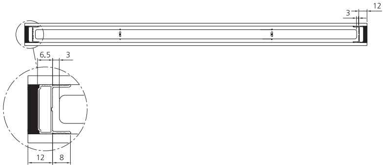
Extrudovaný "C" profil boční vedení 22 x 6.5 mm
