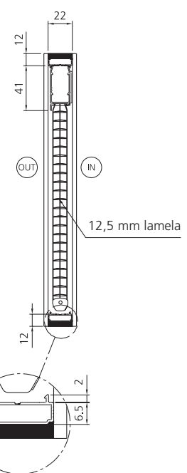
Extrudovaný "U" profil 22 x 6.5 mm
