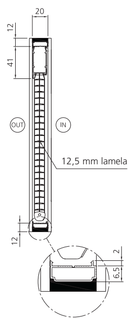
Extrudovaný "U" rámeček 20 x 6.5 mm
