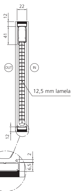
Extrudovaný "U" profil 22 x 6.5 mm
